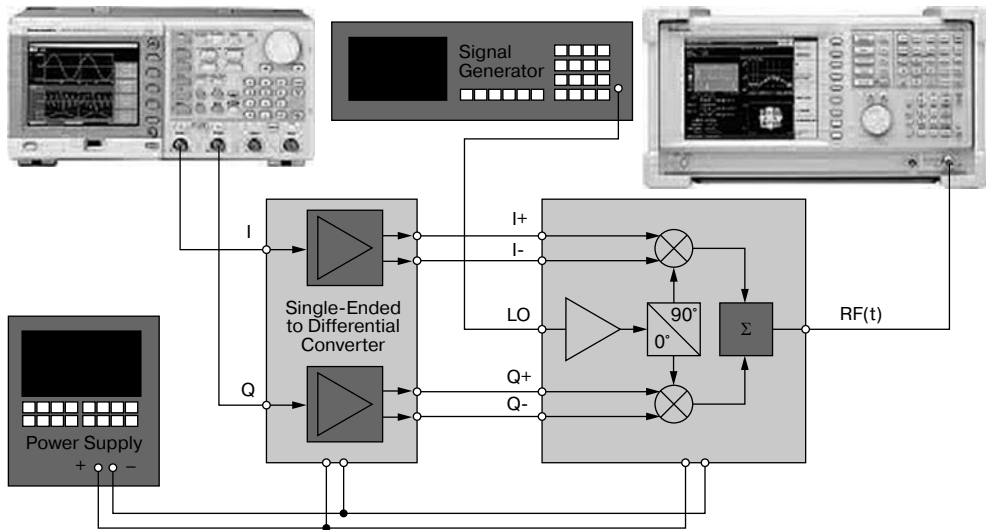
Рис. 5.61. Функциональная схема модели передатчика с QPSK модуляцией
