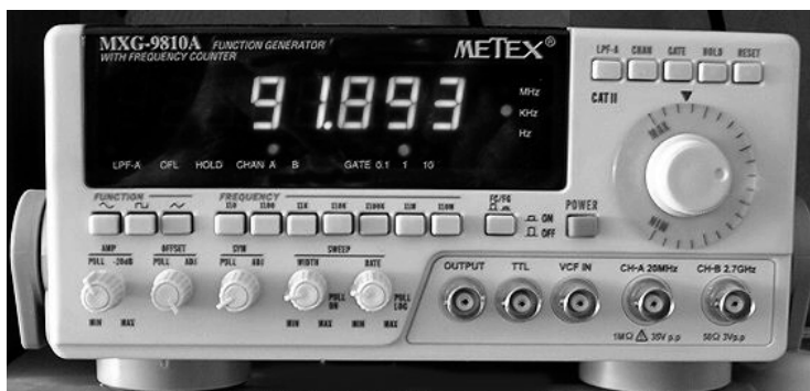
Рис. 3.28. Функциональный генератор и цифровой частотомер MSG-9810A
