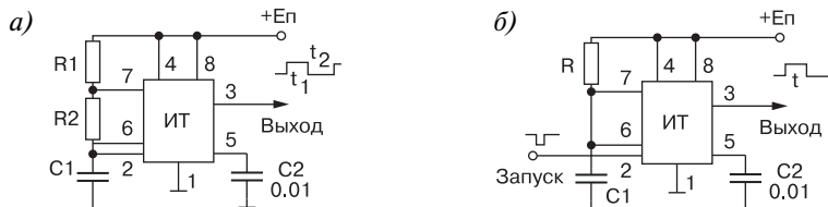
Рис. 2.5. Типовые схемы автоколебательного (а) и ждущего (б) импульсных генераторов (релаксаторов) на интегральном таймере
