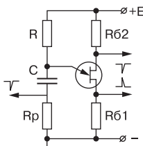
Рис. 2.8. Автоколебательный генератор (релаксатор) на ОПТ
