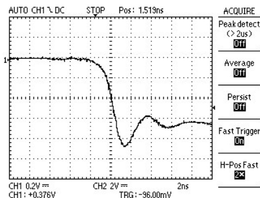
Рис. 5.34. Реакция 250 МГц осциллографа DS-1250 фирмы EZ Digital на отрицательный перепад
