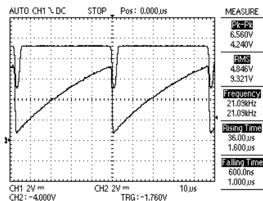
Рис. 2.9. Осциллограммы импульсов на базе 2 (сверху) и на конденсаторе C
