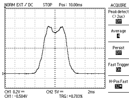
Рис. 5.43. АЧХ двухкантового полосового фильтра промежуточной частоты (копия экрана цифрового осциллографа DS-1250)
