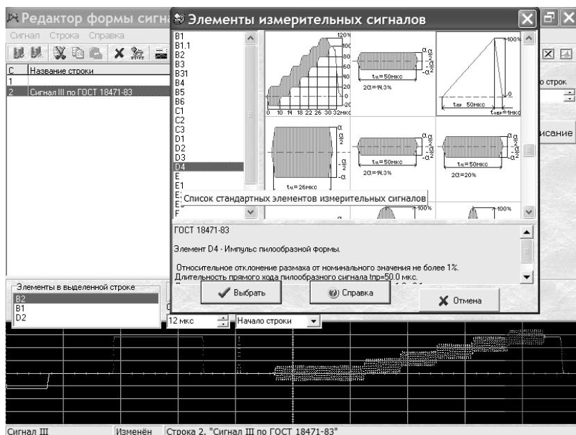
Рис. 2.29. Окно редактора сигналов и окно библиотеки фрагментов сигналов для вставки их в редактируемый сигнал
