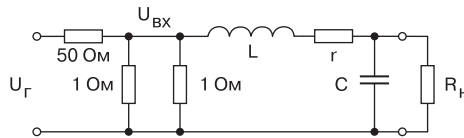
Рис. 5.37. Измерительная схема для измерения параметров LCR-контуров
