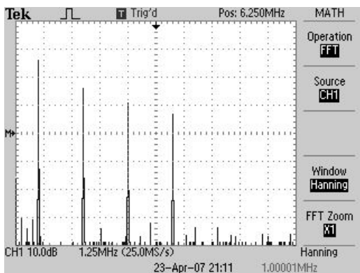
Рис. 4.65. Спектр заданного сигнала, полученный с помощью цифрового осциллографа TDS2124B, при использовании окна Хэннинга
