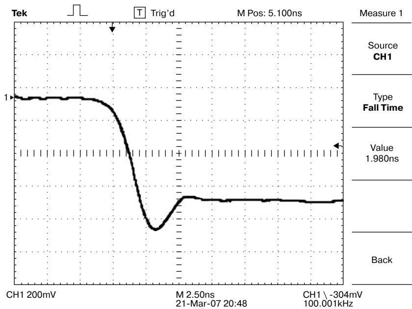
Рис. 5.32. Реакция 200 МГц цифрового осциллографа TDS 2024B на отрицательный перепад
