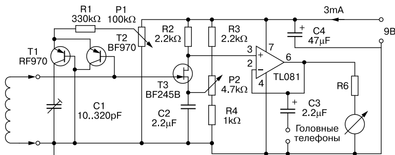
Рис. 1.60. ГИР на транзисторном аналоге негатрона
