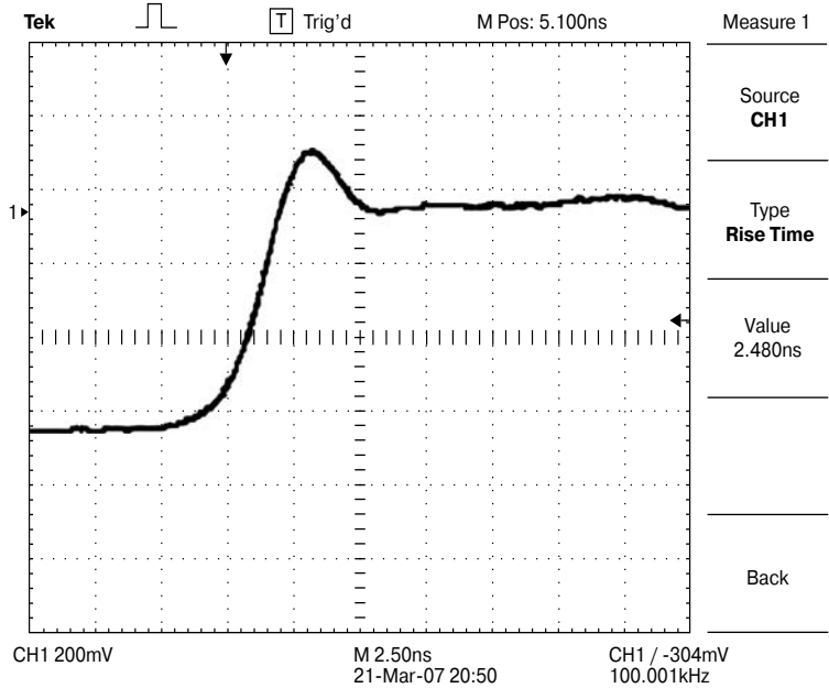
Рис. 5.33. Реакция 200 МГц цифрового осциллографа TDS 2024B на положительный перепад
