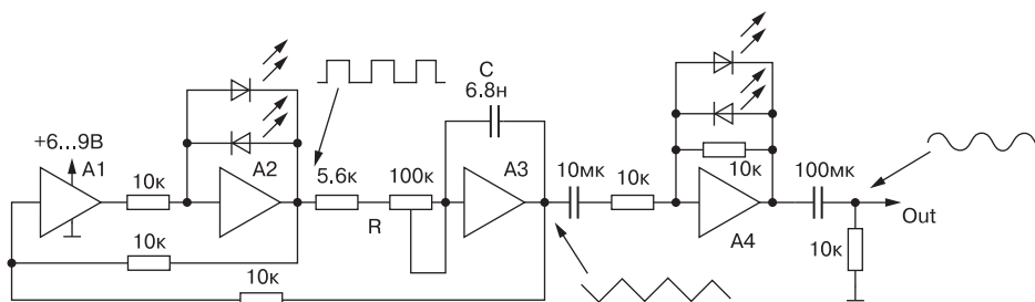
Рис. 3.2. Простая схема функционального генератора на интегральных операционных усилителях
