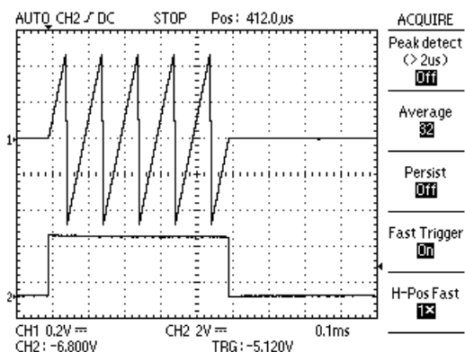
Рис. 4.25. Осциллограммы пачки пилообразных импульсов на основном выходе (верхняя кривая) и импульсов на TTL-выходе запуска (нижняя кривая)
