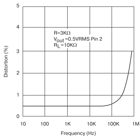
Рис. 3.14. Зависимость коэффициента гармоник синусоидального напряжения от частоты
