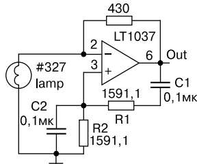
Рис. 1.7. Типичная схема RC -генератора на операционном усилителе
