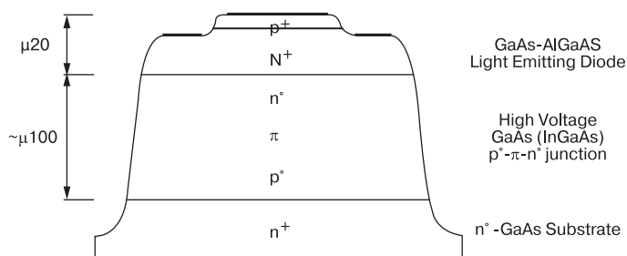
Рис. 2.47. Структура фотоно-ионного инжекционного коммутатора
