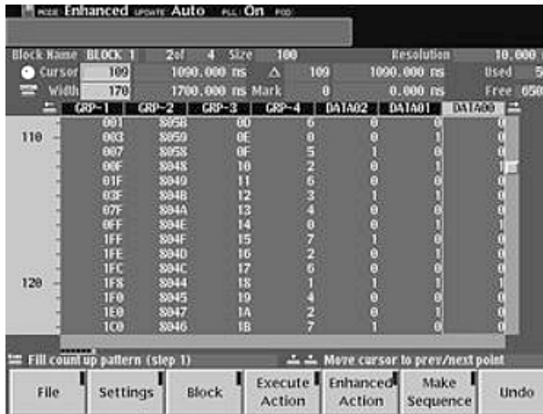
Рис. 4.76. Вид экрана генератора DG2020A в режиме просмотра и редактирования шестнадцатеричного HEX-кода. Диаграммы можно создавать различными способами, в том числе и их программированием с использованием для этого операторов переходов и циклов.
