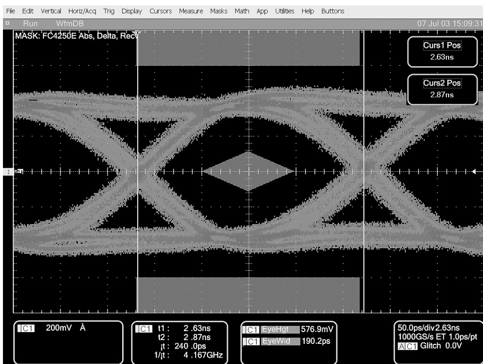
Рис. 5.66. Глазковая диаграмма
