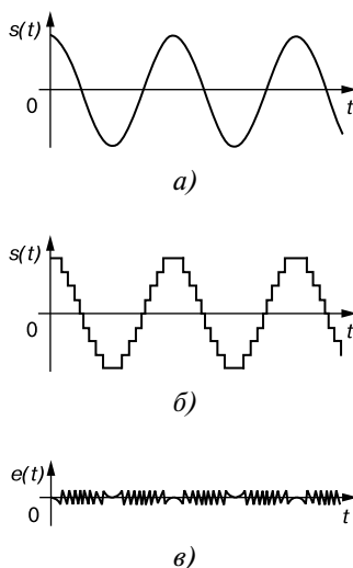
Рис. 1.30. Идеальный синусоидальный сигнал (а), реальный сигнал на выходе ЦАП с запоминанием (б) и шум квантования (в)
