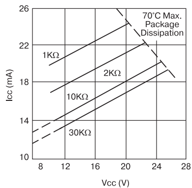
Рис. 3.13. Зависимость потребляемого микросхемой XR-2206 тока от напряжения питания при разных значениях R
