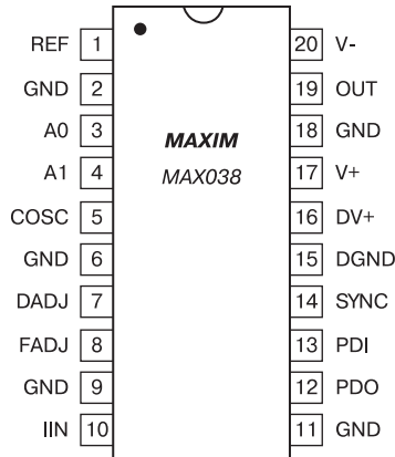
Рис. 3.16. Микросхема MAX038 фирмы MAXIM (вид сверху)
