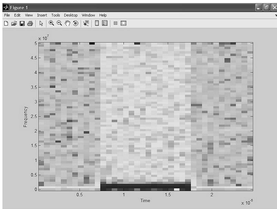
Рис. 4.59. Спектрограмма радиоимпульса
