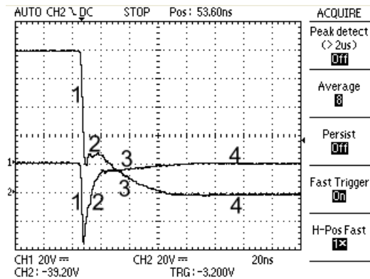
Рис. 2.15. Осциллограммы импульсов разрядного тока и напряжения на коллекторе лавинного транзистора 2Т312В
