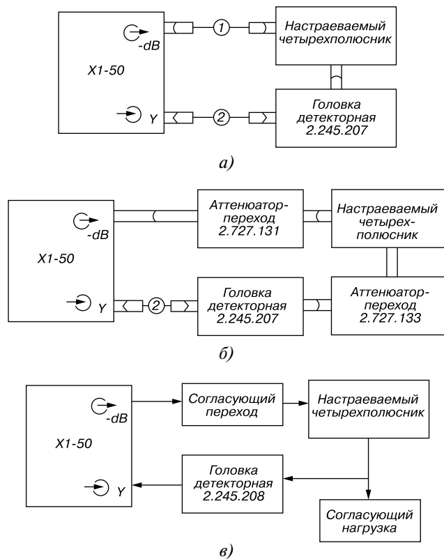
Рис. 1.57. Основные функциональные схемы применения измерителя АЧХ X1-50:
