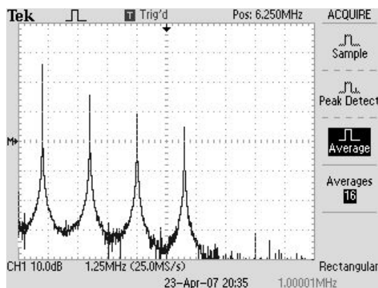
Рис. 4.64. Спектр заданного сигнала при прямоугольном окне, полученный с помощью цифрового осциллографа TDS2124B
