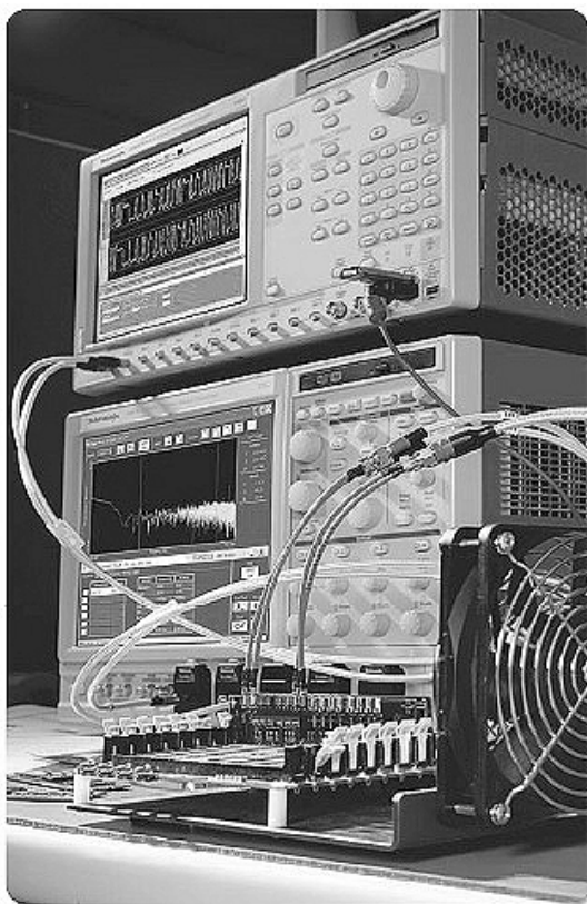
Рис. 5.70. Приборы на рабочем месте испытания и тестирования UBW-устройств
