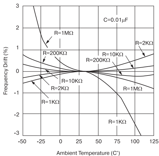
Рис. 3.15. Изменение частоты при изменении температуры для схемы генератора с рис. 3.11 при различных R
