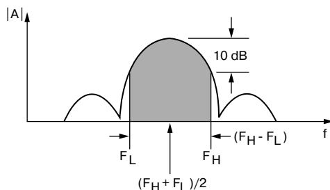
Рис. 5.68. Спектр UWB-систем
