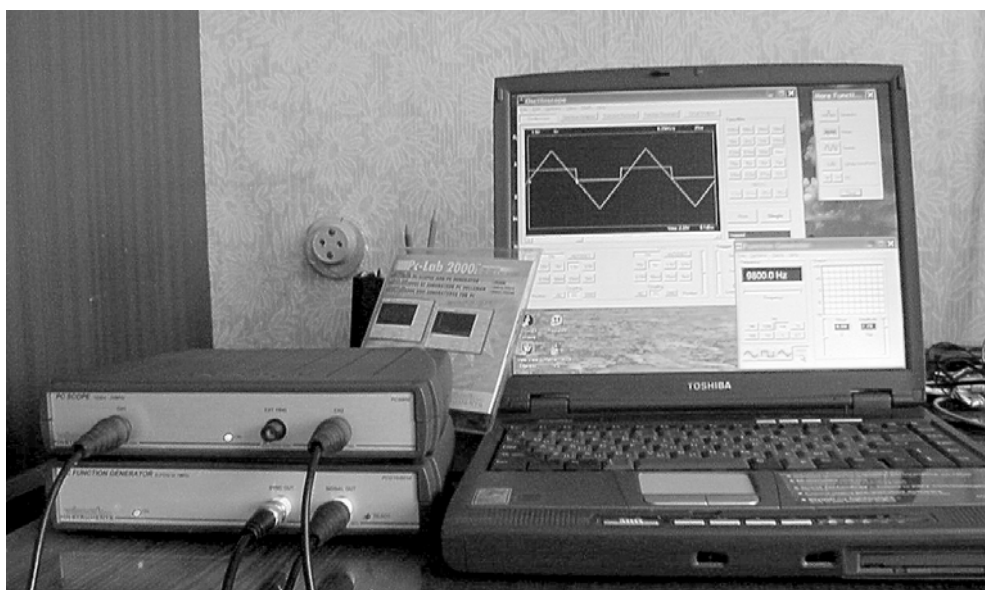
Рис. 3.53. Внешний вид компьютерной измерительной системы на базе виртуальных приборов и мобильного компьютера — ноутбука Satellite 1800-314 корпорации Toshiba
