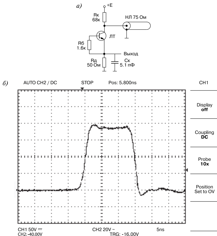
Рис. 2.16. Генератор прямоугольных импульсов на лавинном транзисторе КТ630А с накопительной линией в виде отрезка коаксиального кабеля (а) и осциллограмма выходного импульса при E_n = 300 В (б)
