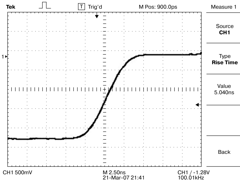
Рис. 5.26. Передний фронт импульсов генератора AFG3101 (осциллограмма получена с помощью осциллографа TDS 2024B фирмы Tektronix)
