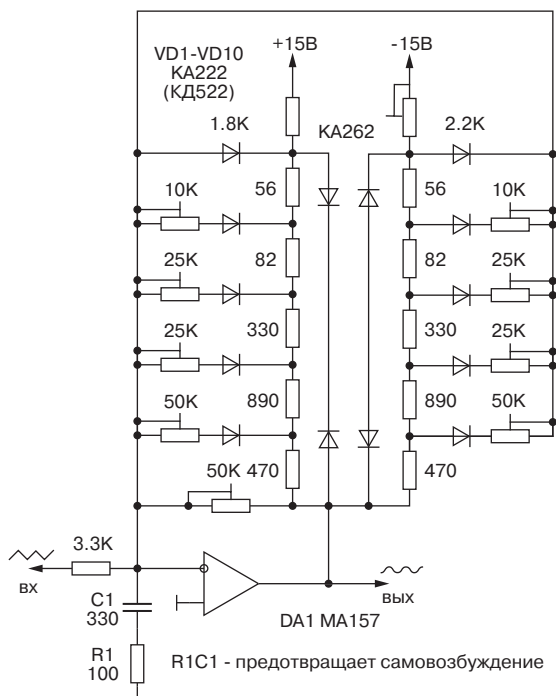
Рис. 3.7. Формирователь синусоидального сигнала из треугольного с 5-уровневым ограничителем
