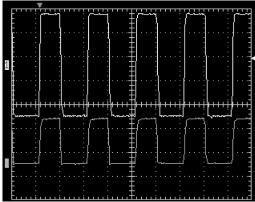
Рис. 3.30. Осциллограммы прямоугольного и TTL сигналов на частоте 1 МГц
