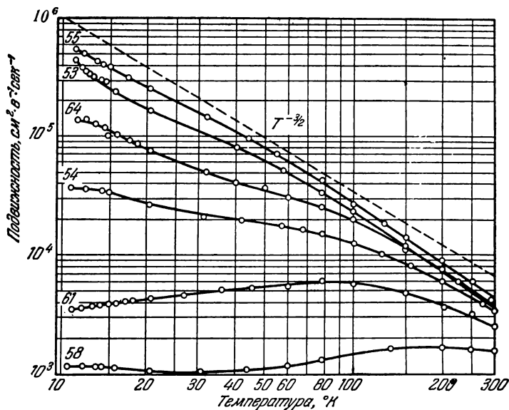
Рис. 7.10. Температурная зависимость подвижности для того же, что и на рис. 7.8 и 7.9 ряда кристаллов германия с примесями мышьяка. Пунктирная линия соответствует теоретической зависимости по закону T^{-3/2} для абсолютно чистого кристалла, когда подвижность ограничивается только рассеянием на решетке (по Конуэлл).
