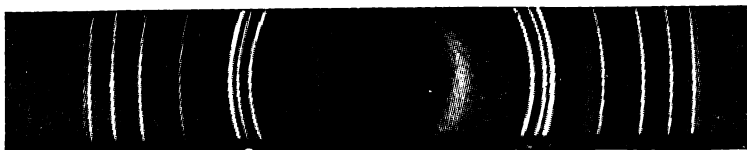
Рис. 2.11. Порошковая рентгенограмма (дебаеграмма), полученная на кристаллах \text{ZnO} .
