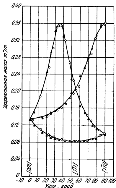
Рис. 7.15. Зависимость эффективной массы электронов в германии при 4° К от угла между направлением магнитного поля, лежащего в плоскости (110), и осью [001]. Теоретические кривые построены для m_l = 1,58m и m_t = 0,082m . (Из работы [7].)
