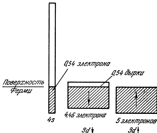
Рис. 6.26. Схемы энергетических зон в никеле при абсолютном нуле.
