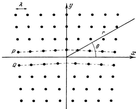
Рис. 9.4. Структура краевой дислокации. Можно считать, что деформация вызвана появлением лишней атомной плоскости, совпадающей на рисунке с верхней половиной оси y . В верхней половине кристалла ( P ) имеет место сжатие, в нижней половине ( Q ) — растяжение. Такая дислокация называется положительной. Если лишняя атомная плоскость проходит в нижней половине кристалла, то дислокация называется отрицательной (по Коттрелу).
