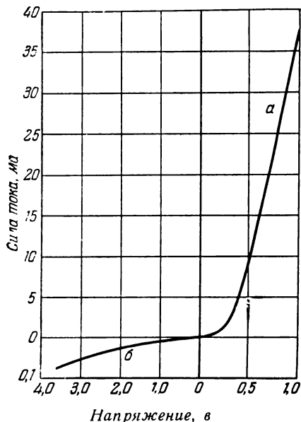
Рис. 7.19. Вольтамперная характеристика выпрямителя из окиси меди а — прямой ток; б — обратный ток. (Масштаб по осям в обе стороны от начала координат — различный.)
