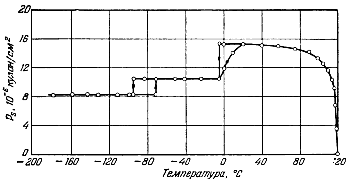
Рис. 4.14. Зависимость самопроизвольной поляризации титаната бария от температуры.
