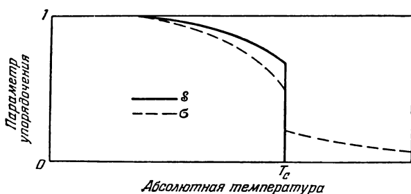
Рис. 6.33. Зависимость от температуры параметров дальнего ( s ) и ближнего ( \sigma ) порядка для сплава типа AB_3 (из статьи Никса и Шокли [15]).
