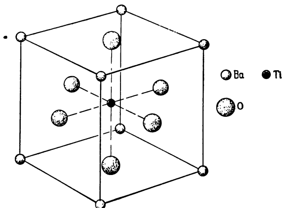
Рис. 4.11. Структура типа перовскита, свойственная титанату бария.
