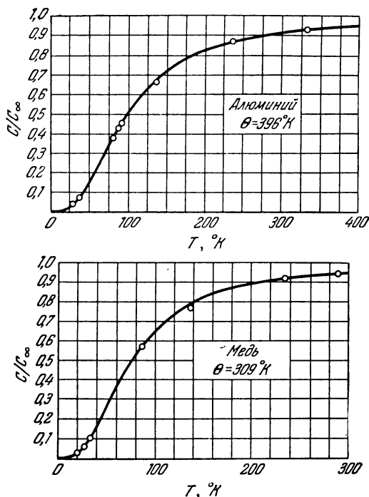
Рис. 3.4. Теплоемкость алюминия и меди как функция температуры. Кривые построены на основе теории Дебая, причем для алюминия взято \theta = 396^\circ K , для меди \theta = 309^\circ K . Кружками показаны экспериментальные данные (из работы Дебая [7]).
