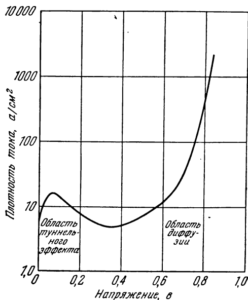
Рис. 7.27. Вольтамперная характеристика кремниевого туннельного диода при наложении напряжения в прямом направлении (по Эсаки).
