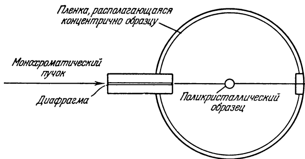
Рис. 2.10. Схема устройства камеры, используемой в порошковом методе.
