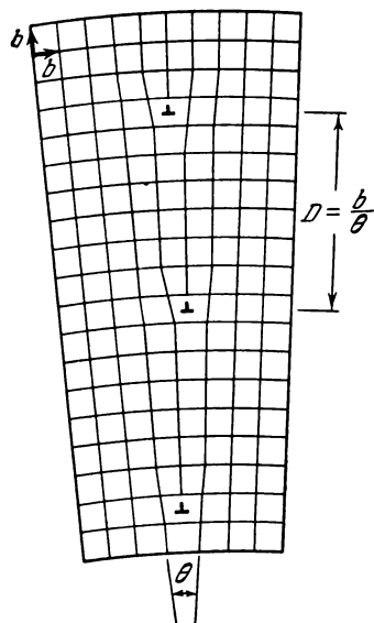
Рис. 9.9. Граница зерен с малым углом разориентировки (по Бюргерсу). Значок \perp указывает положения краевых дислокаций. Верхним своим концом значок указывает положение лишней атомной плоскости.
