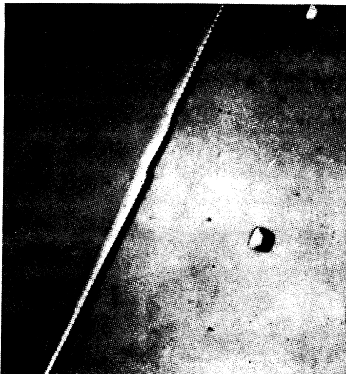
Рис. 9.10. Ямки травления на поверхности (100) образца германия вдоль границы с малым углом разориентировки. Угол между кристаллитами равен 27,5 угловой секунды. Граница лежит в плоскости (0\bar{1}1) . Направление линии дислокации совпадает с направлением [100] . Вектор Бюргерса в данном случае является кратчайшим из векторов трансляции решетки, а именно
