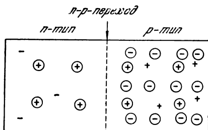
Рис. 7.23. Образование p-n -перехода путем создания области p -типа введением избыточного количества акцепторной примеси, подавляющей доноры и создающей p -проводимость.
