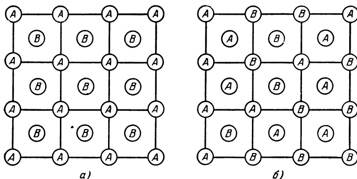
Рис. 6.32. Упорядоченное (а) и неупорядоченное (б) расположение ионов A и B в сплаве AB .
