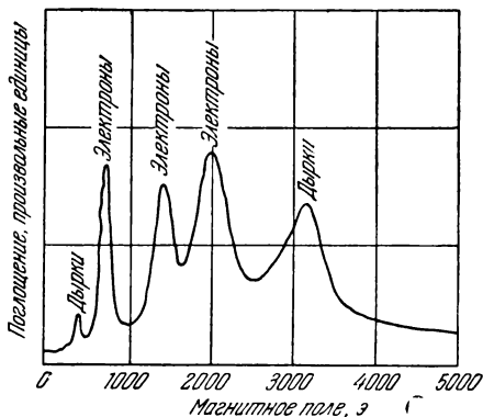
Рис. 7.14. Типичная кривая циклотронного резонансного поглощения, полученная на кристалле германия при T = 4^\circ\text{K} вблизи частоты 24\,000\text{ Мгц} ; кривая представляет собой непосредственное воспроизведение автоматически записанной зависимости поглощаемой мощности от величины статического поля, расположенного в плоскости (110) кристалла под углом 60^\circ к оси [100].
