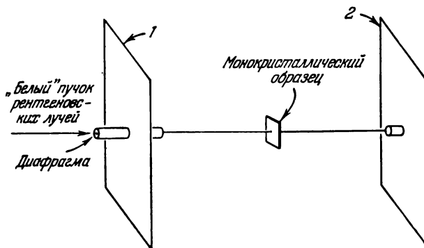
Рис. 2.7. Камера, используемая в методе Лауэ.
