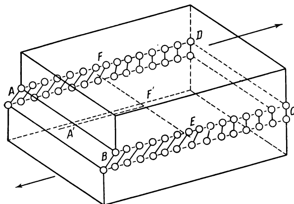
Рис. 9.3. Краевая дислокация в плоскости скольжения ABCD . В области ABEF атомы смещены более чем на половину постоянного расстояния решетки; в области FECD атомы смещены менее, чем на половину постоянного расстояния решетки; EF — линия дислокации, A'F' — направление скольжения (по Коттрелу [2]).
