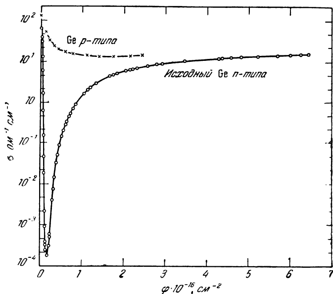
Рис. 7.18. Зависимость проводимости образцов германия от величины интегральной дозы облучения дейтронами. Один из образцов был первоначально материалом n -типа, другой p -типа. (Данные группы университета Пардю.)
