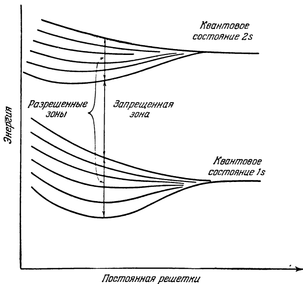
Рис. 6.5. Образование энергетических уровней в системе из шести водородных атомов при их сближении (т. е. при уменьшении постоянной решетки).
