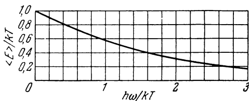
Рис. 3.2. Зависимость средней энергии эйнштейновского осциллятора от частоты [средняя энергия и частота (умноженная на \hbar ) отнесены к kT ].
