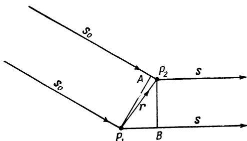
Рис. 2.2. К вычислению разности фаз волн, рассеянных двумя точками решетки.
