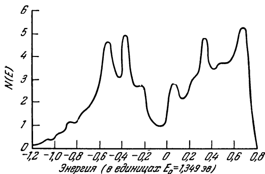
Рис. 6.29. Плотность состояний N(E) в d -зонах никеля как функция энергии E (в единицах E_0 = 1,349 эв). (Из работы Костера [14].)
