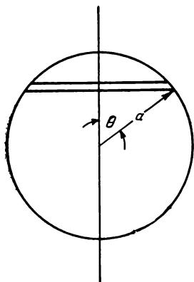
Рис. 4.3. К расчету поля в сферической полости внутри однородно поляризованной среды. Заряд кольца равен 2\pi a \sin \theta a d\theta P \cos \theta .
