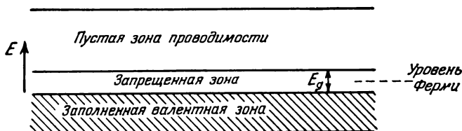
Рис. 7.1. Схема энергетических зон, поясняющая явление собственной проводимости.
