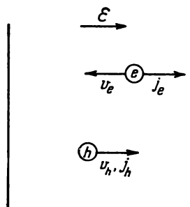
Рис. 7.2. Движение электронов ( e ) и дырок ( h ) в электрическом поле \mathcal{E} . Показаны направления скорости ( v ) и тока ( j ).
