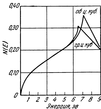
Рис. 6.23. Число состояний N(E) на единичный энергетический интервал, как функция энергии для гранецентрированной и объемноцентрированной кубических решеток.
