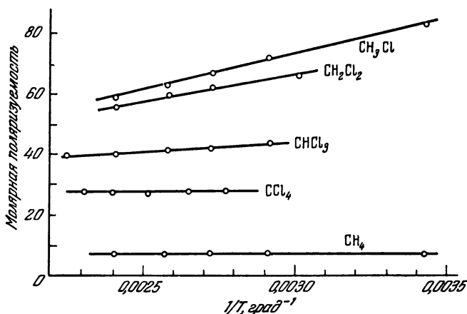
Рис. 4.7. Величина (M/\rho)(\epsilon - 1)/(\epsilon + 2) = 4\pi L a/3 (называемая молярной поляризуемостью) как функция обратной температуры для соединений полярного и неполярного замещенного метана в газообразном состоянии [9].
