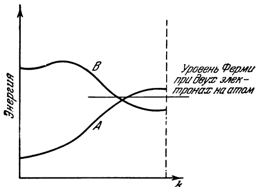
Рис. 6.6. Схематическое изображение перекрывания зон A и B , которое может иметь место в кристаллах двухвалентных элементов и приводить к металлической проводимости.
