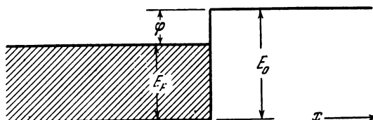
Рис. 5.8. К расчету термоэлектронной эмиссии.
