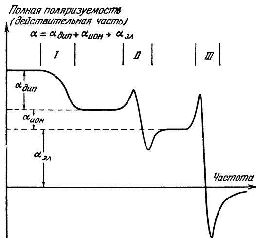
Рис. 4.6. Схематическая кривая, иллюстрирующая частотную зависимость различных составляющих действительной части полной поляризуемости.
