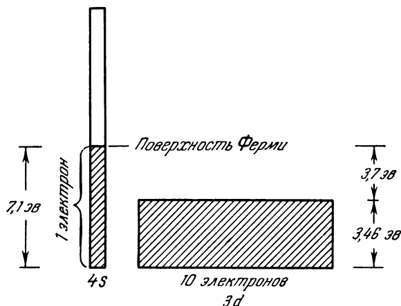
Рис. 6.24. Схема энергетических 4s- и 3d-зон в металлической меди.
