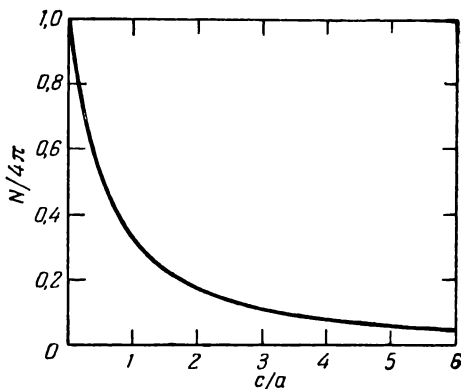
Рис. 4.2. Кривая зависимости деполяризующего фактора в направлении оси симметрии эллипсоида вращения от величины отношения осей c/a .
