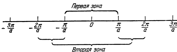
Рис. 6.13. Зоны Бриллюэна для линейной решетки из одинаковых атомов с постоянной решетки, равной a .
