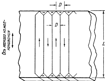
Рис. 8.19. Расположение замыкающих доменов в магнитно-одноосном кристалле.
