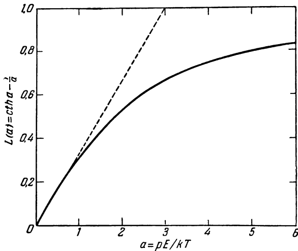
Рис. 4.8. Кривая зависимости функции Ланжевена L(a) от своего аргумента a = pE/kT .
