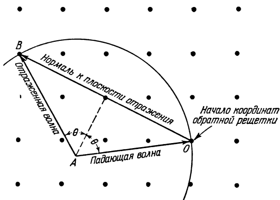
Рис. 2.4. Построение Эвальда в обратной решетке.
