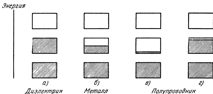
Рис. 6.1. Схематическое изображение заполненности электронами разрешенных энергетических зон для изолятора, металла и двух полупроводников.
