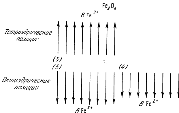
Рис. 8.23. Схема спинового расположения в магнетите \text{FeOFe}_2\text{O}_3 , иллюстрирующая компенсацию моментов ионов \text{Fe}^{3+} (магнитный момент иона \text{Fe}^{3+} равен 5\mu_B ). Результирующая намагниченность создается магнитными моментами ионов \text{Fe}^{2+} , которые остаются нескомпенсированными. Каждый ион \text{Fe}^{2+} имеет магнитный момент, равный 4\mu_B ; поскольку на ячейку приходится восемь таких ионов, то намагниченность на ячейку должна быть равна 8 \cdot 4\mu_B = 32 \mu_B , измерения же дают 8 \cdot 4,0 \cdot 7 \mu_B = 32,56 \mu_B .
