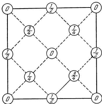
Рис. 1.10. Расположение атомов в элементарной ячейке структуры алмаза (проекция на грань куба).
