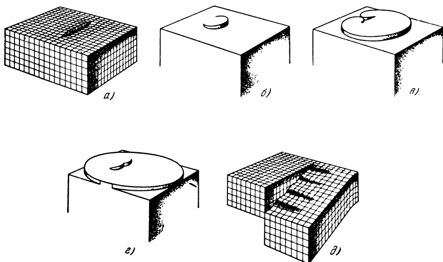
Рис. 9.16. Ступенька роста в виде замкнутой петли a) может возникнуть из ступеньки, которая начинается и кончается в пределах верхней грани кристалла, соединяя выходы двух винтовых дислокаций разных знаков. Такая ступенька закреплена на обоих концах и может дать начало росту следующего слоя. На рис. б) показан первый этап роста — образование округленной ступеньки на поверхности кристалла; далее на рис. в) видно, как закругленные «края» ступеньки сомкнулись позади ее исходного положения. В конечном итоге (рис. г) ) внутренний участок сомкнется (зарастет) и над ним поднимется новая ступенька, такая же, как и исходная. На рис. д) изображена четырехслойная ступенька, образованная четырьмя близко расположенными дислокациями одного знака. Большие группы дислокаций дают многослойные ступеньки.
