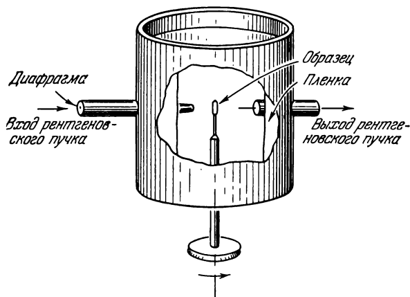
Рис. 2.9. Камера, используемая в методе вращения кристалла [1].
