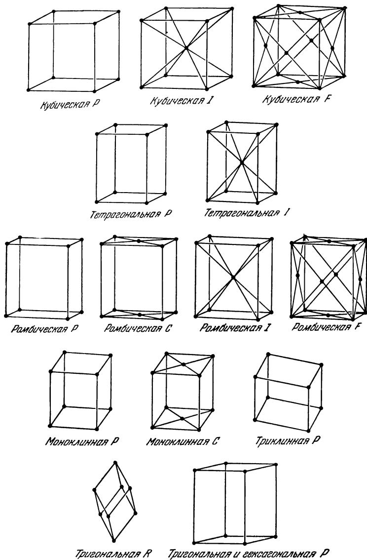
Рис. 1.4. Четырнадцать решеток Браве, называемых также пространственными решетками.
