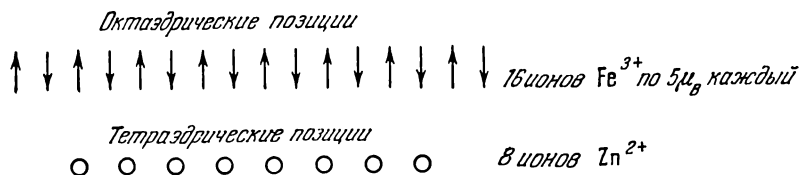
Рис. 8.26. Схема расположения магнитных моментов в цинковом феррите, объясняющая, почему намагниченность насыщения цинкового феррита равна нулю. Ионы цинка диамагнитны и занимают тетраэдрические позиции (см. рис. 8.27). Магнитная структура этого феррита характеризуется антиферромагнитным расположением ионов железа в октаэдрических позициях.
