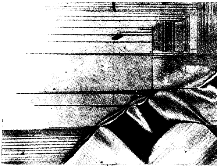
Рис. 4.18. Клинообразные пластинчатые домены в монокристалле титаната бария (из работы Форсберга [29]).
