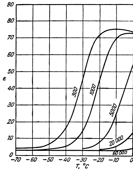
Рис. 4.9. Температурная зависимость диэлектрической проницаемости льда при различных частотах (значения частоты в герцах приведены у кривых). (Из работы Смита и Хичкока [10].)
