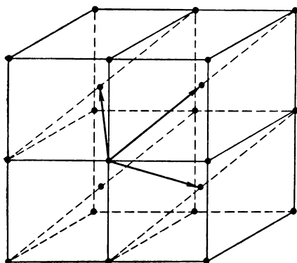
Рис. 1.5. Векторы основных трансляций в объемноцентрированной кубической решетке. Примитивная ячейка получается дополнением до ромбоэдра.
