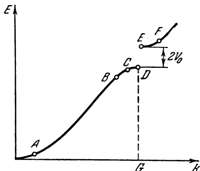
Рис. 6.8. Зонная структура, вызванная возмущающим потенциалом вида 2V_0 \cos Gx .
