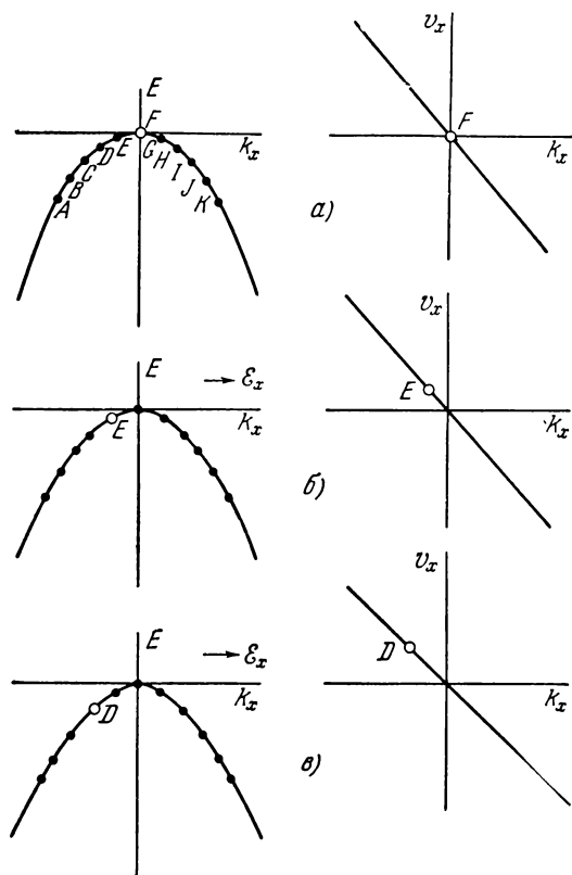
Рис. 6.10. а) При t = 0 все состояния заняты, за исключением состояния F в вершине зоны; б) электрическое поле \mathcal{E}_x наложено в положительном направлении оси x . На электрон действует сила в направлении -k_x , и все электроны одновременно перемещаются вправо, так что вакантное состояние (дырка) смещается влево и занимает позицию E ; в) дальнейшее перемещение электрона сдвигает дырку еще дальше влево, и она занимает позицию D . Таким образом, дырка перемещается в направлении уменьшения значений k_x , соответствующих большим положительным скоростям.
