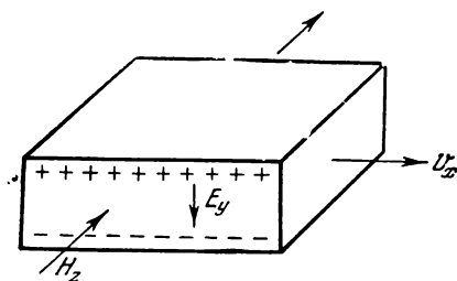
Рис. 6.11. Эффект Холла.
