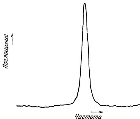
Рис. 8.5. Протонное спиново-резонансное поглощение в растворе азотнокислого железа (постоянное магнитное поле фиксировано, частота изменяется) (из работы [3]). В поле 7050 э резонанс наступает при частоте 30 МГц.
