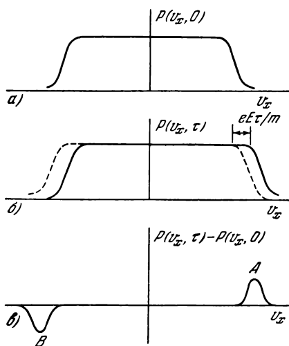
Рис. 5.7. Распределение скоростей в случае статистики Ферми — Дирака (одномерный случай).
