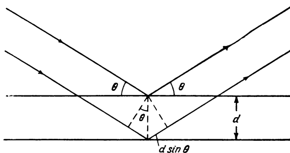
Рис. 2.1. К выводу формулы Брэгга: 2d \sin \theta = n\lambda , где d — расстояние между атомными плоскостями; 2\pi n — разность фаз между отражениями от следующих плоскостей.
