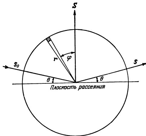
Рис. 2.5. К расчету атомного фактора рассеяния f . Вектор \mathbf{S} является нормалью к плоскости рассеяния.
