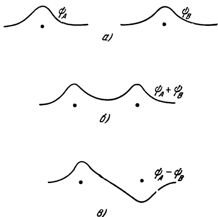
Рис. 6.4. а—волновые функции электронов в двух водородных атомах, расположенных далеко друг от друга; б—линейная комбинация этих волновых функций, описывающая состояние сближенных атомов; в—линейная комбинация, описывающая возбужденное состояние.
