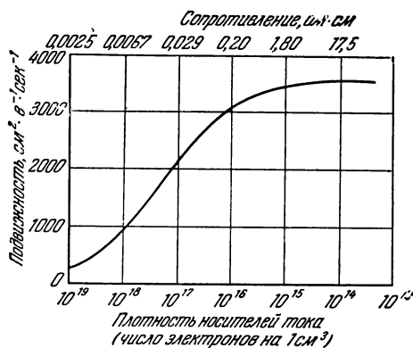
Рис. 7.7. Теоретическая кривая зависимости подвижности от плотности носителей тока в германии n -типа при 300^\circ \text{K} . Нижняя шкала (плотность) — число электронов в 1 \text{ см}^3 , верхняя — сопротивление (в \text{ом} \cdot \text{см} ). Предполагается, что все донорные атомы ионизованы, а акцепторы отсутствуют (по Конуэлл).
