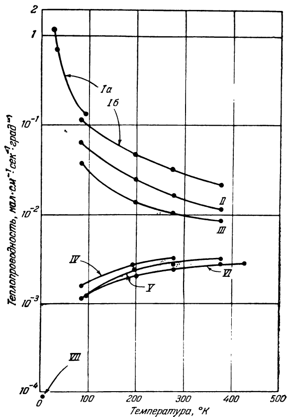
Рис. 3.6. Температурная зависимость теплопроводности ряда кристаллов и стекол.
