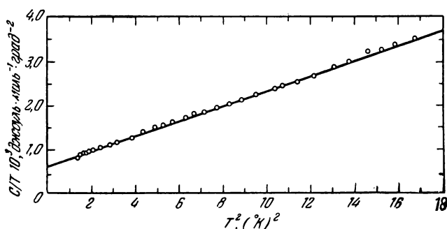
Рис. 3.5. Теплоемкость металлического серебра (по данным Корака, Гарфункеля, Саттеруэйта и Векслера).
