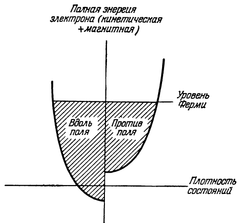
Рис. 5.5. Парамагнетизм Паули при 0^\circ \text{K} .
