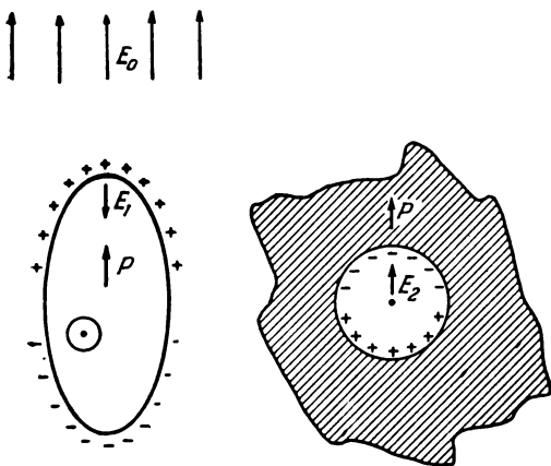
Рис. 4.1. Схематическое изображение полости внутри диэлектрика, поясняющее роль различных факторов, формирующих поле внутри диэлектрика, действующее на ион, расположенный в центре такой полости.
