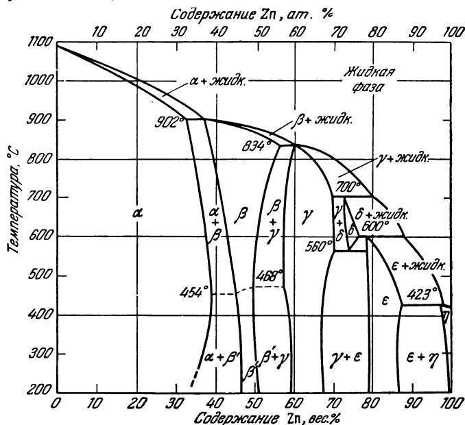
Рис. 6.22. Фазовая диаграмма сплава Cu—Zn.
